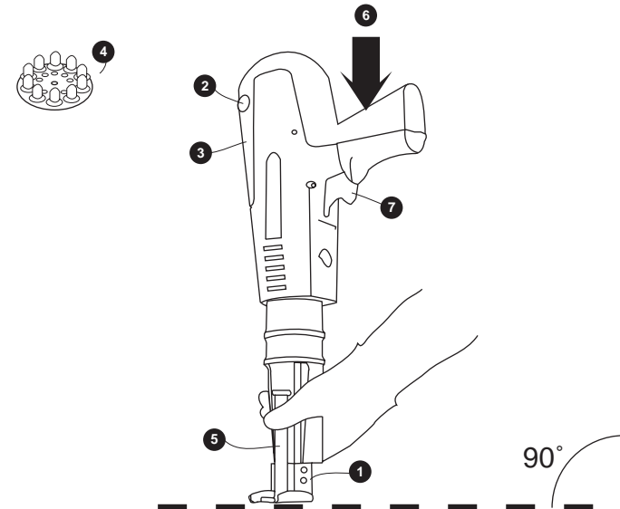
CONECTOR TECNARIA PARA FIJACIÓN POR DISPARO con clavos premontados
